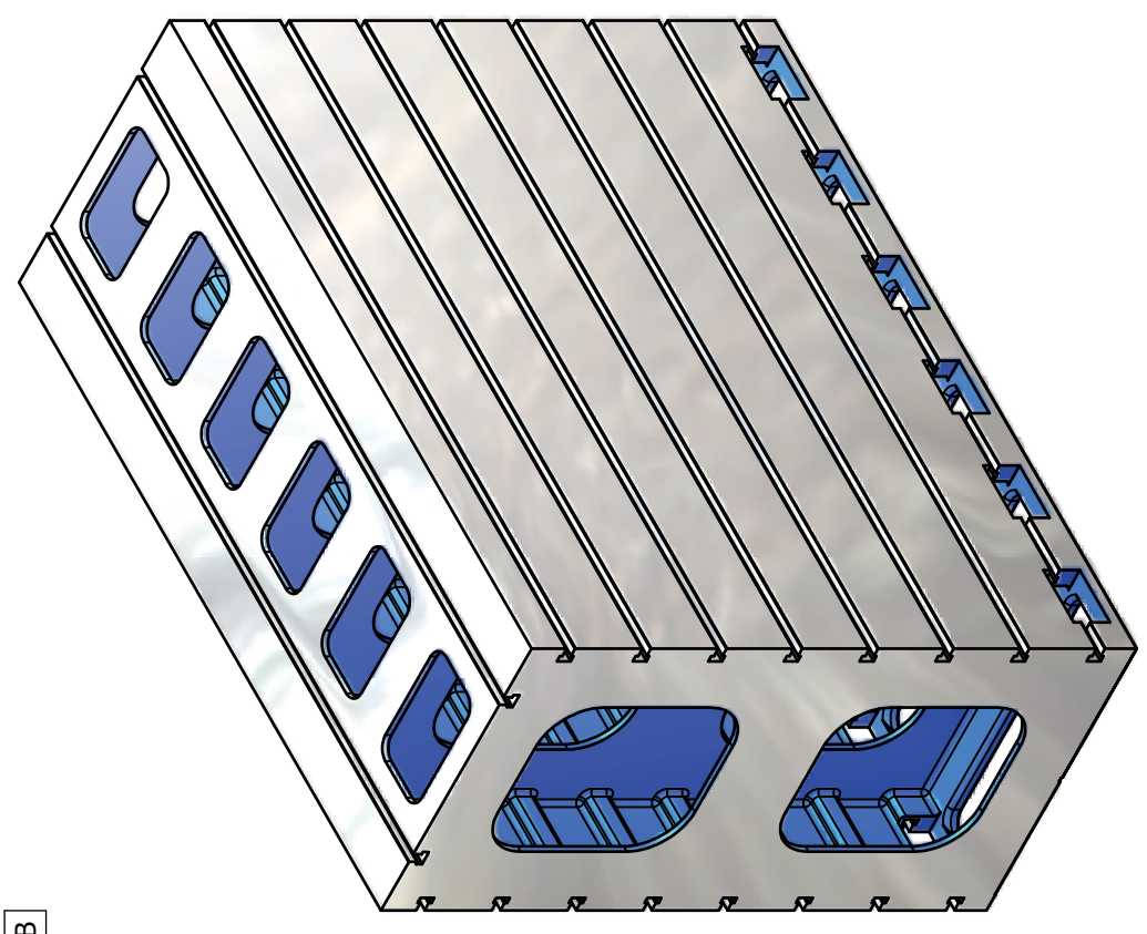
Clamping cube E 4 Upínací kostka E 4
